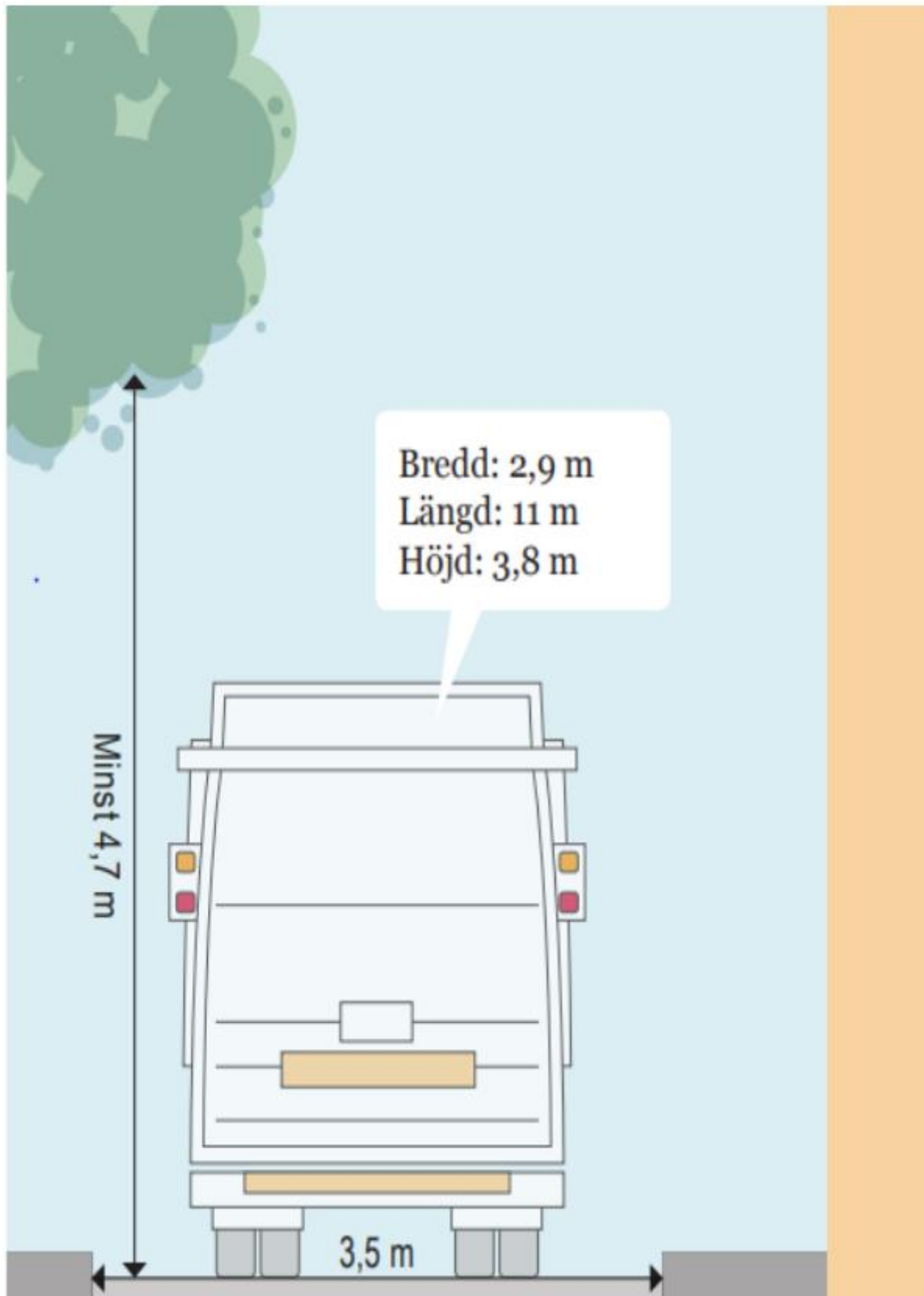
Figur 1 Måttangivelser för fordon
